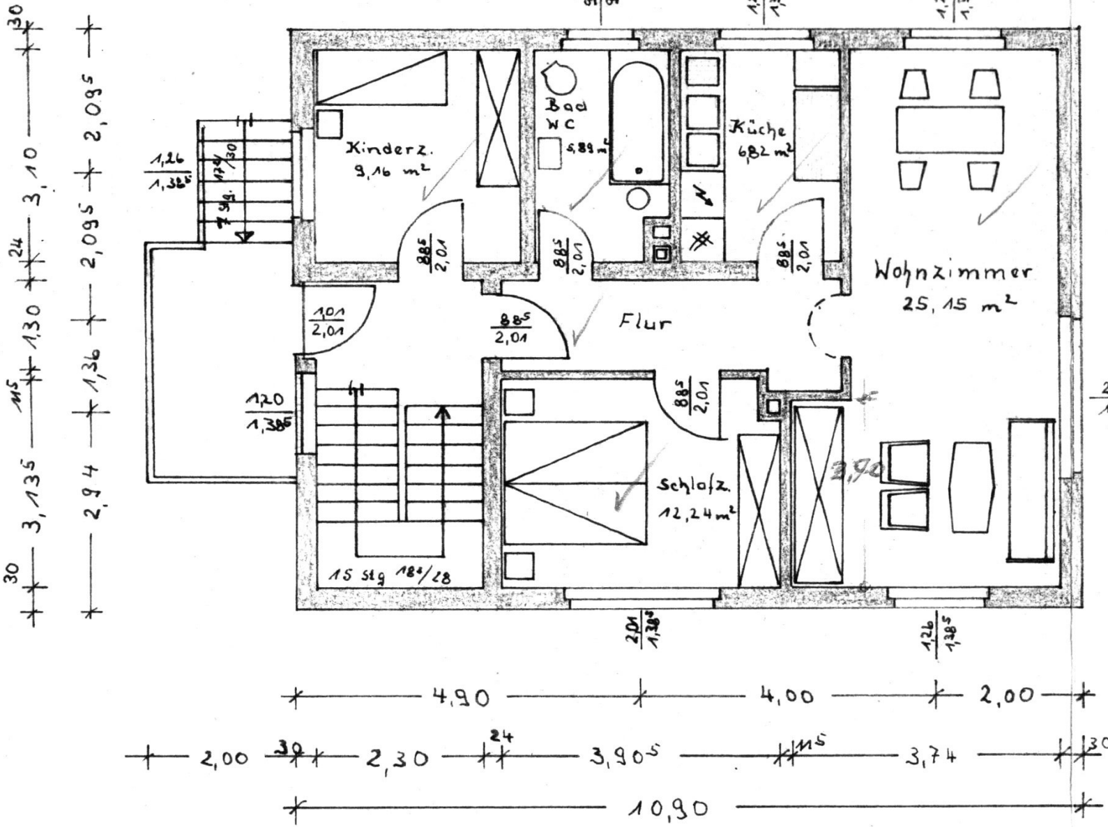
Erdgeschoss
